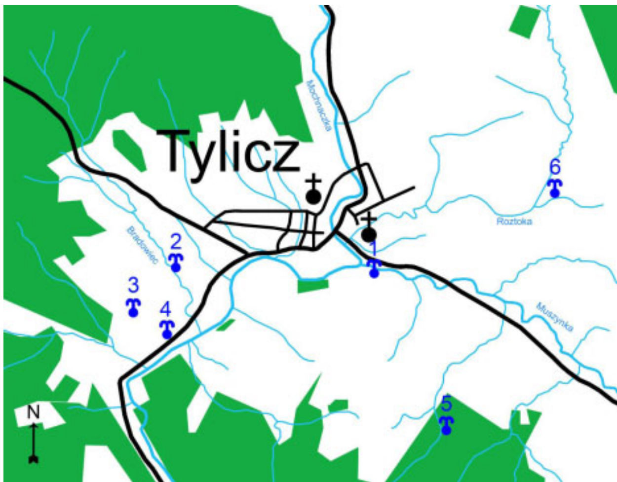
Wody mineralne Tylicza: 1 – Pijalnia Tyliczanka, Zdrój Główny, 2 – Pijalnia Bradowiec, 3 – Mofeta Tylicz, 4 – Zdrój Syhowne (Wedrowców), 5 – Źródło Pod Przekąźnikiem, 6 – Mofeta Pod Beskidem
