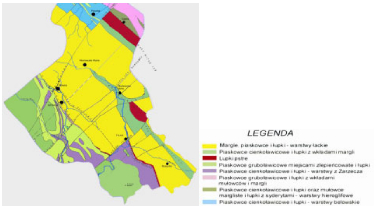
Mapa geologiczna rejonu Krynicy i Tylicza
